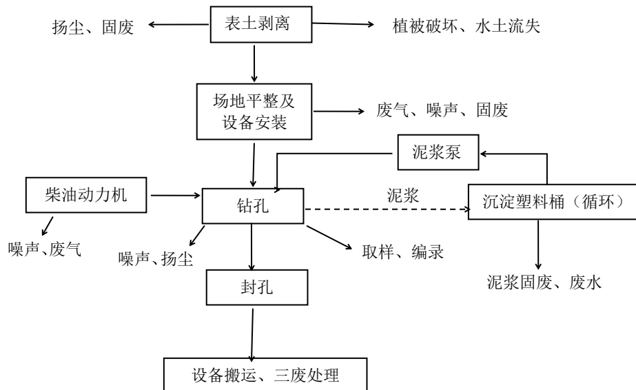
图 2-2 钻探工艺流程及产污环节
